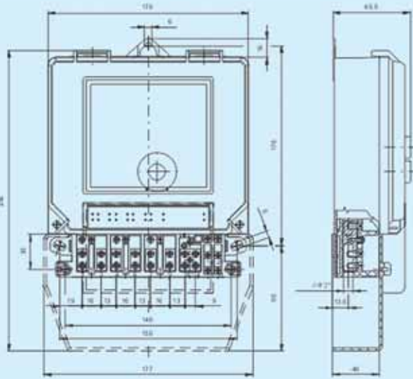
Rozmerový náčrt:
